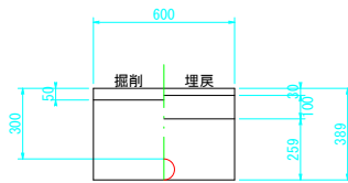
⑫町道 H=0.3m レンタル管80A(設置)
