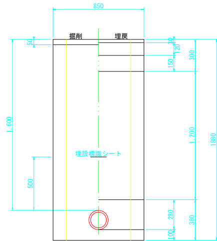
②町道 H=1.6m HPPEφ150
