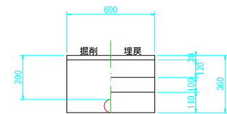
⑮' 町道 H=0.3m PPφ50(撤去)
