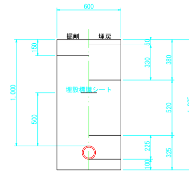
⑧県道 H=1.0m HPPEφ100
