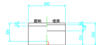
⑮町道 H=0.3m PPφ50(設置)
