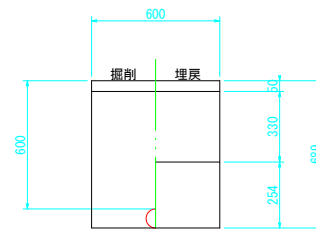
⑭' 県道 H=0.6m レンタル管80A(撤去)
