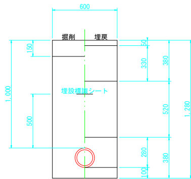
⑥県道 H=1.0m HPPEφ150
