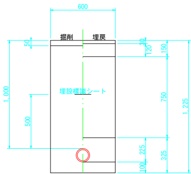
⑤その他町道 H=1.0m HPPEφ100
