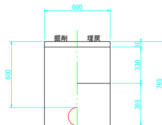
⑬' 県道 H=0.6m レンタル管150A(撤去)
