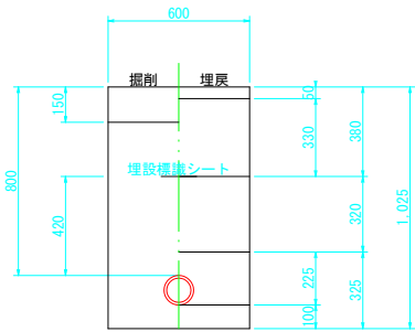
⑩町道 H=1.0m H1VP φ75
