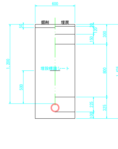
④町道 H=1.2m HPPEφ100
