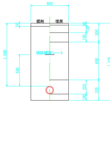
③町道 H=1.0m HPPEφ100
