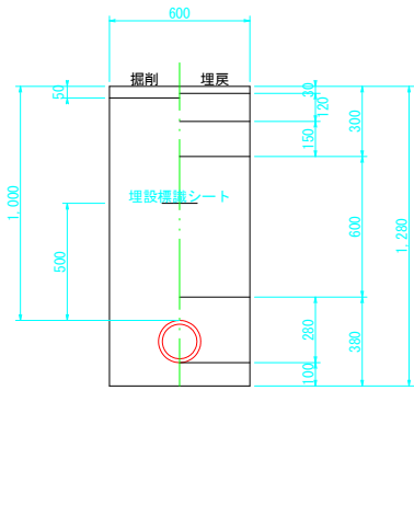
①町道 H=1.0m HPPEφ150
