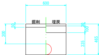
⑪' 町道 H=0.3m レンタル管150A(撤去)
