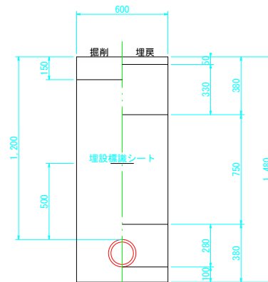
⑦県道 H=1.2m HPPEφ150
